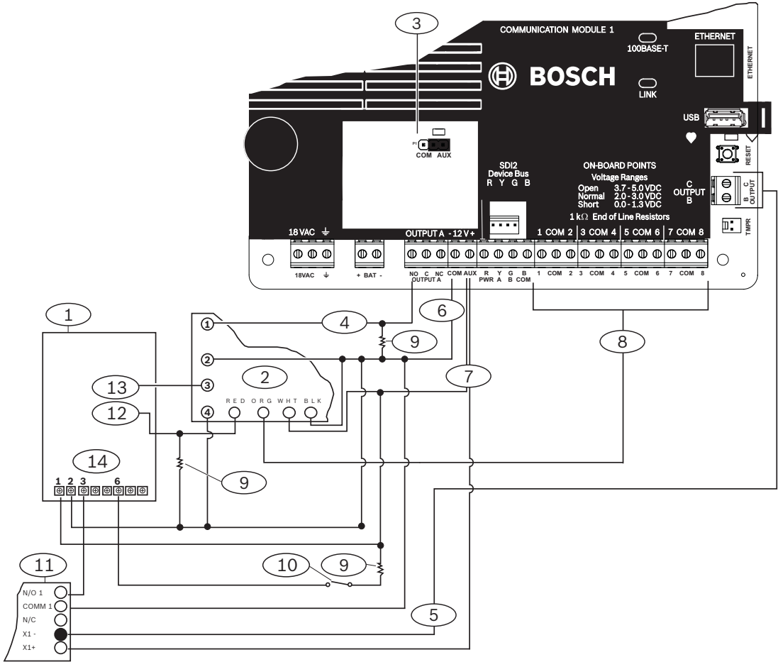
Figura 19.1: Cableado detallado de la sirena de alta seguridad Rothenbuhler 5110_4001-42 al panel de control (se muestra el B5512)
