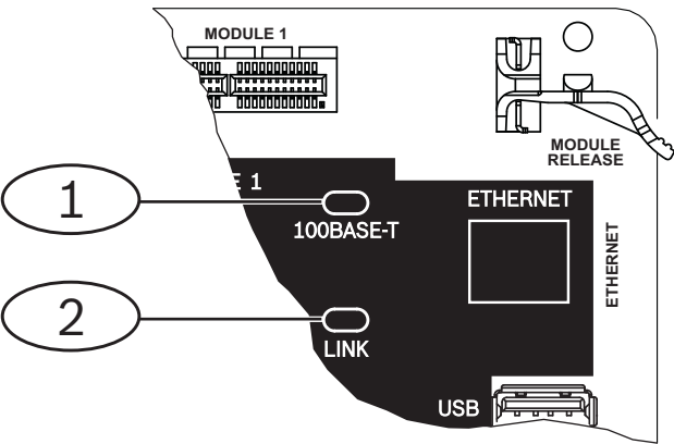
Figura 8.1: Ethernet y LED integrados en placa (se muestra el B5512)
