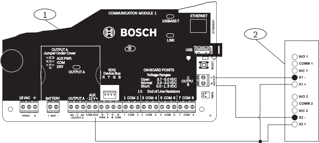
Figura 10.1: Cableado de SALIDA B y C (se muestra el B5512)
