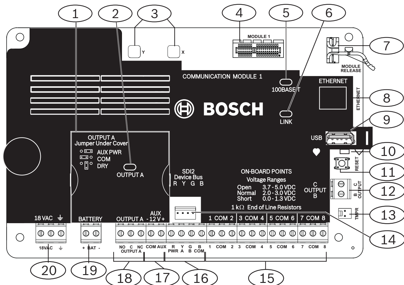
Figura 17.1: Descripción general del módulo del panel de control (se muestra el B5512)
